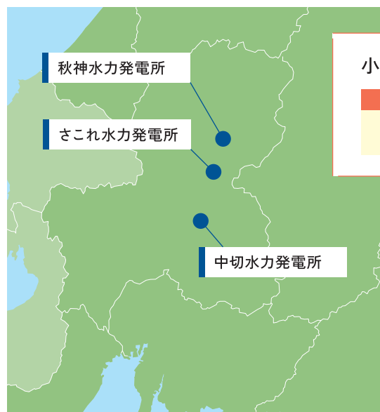
■ 秋神水力発電所
