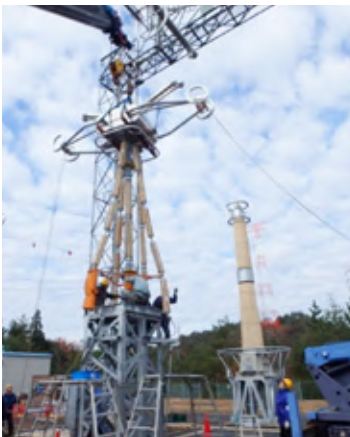
■ 500kV 断路器組立工事
