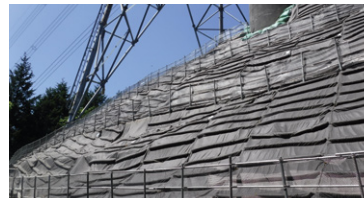
雨水誘導マットによる表層土砂流出対策
