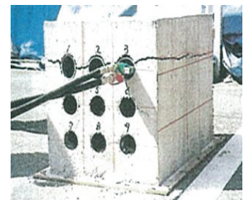
模擬管路による破砕試験
